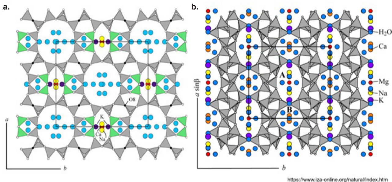
Зураг 1. ЭХС-д түгээмэл хэрэглэгддэг байгалийн цеолит (а. клиноптилолит, б. морденит)-ын бүтэц
