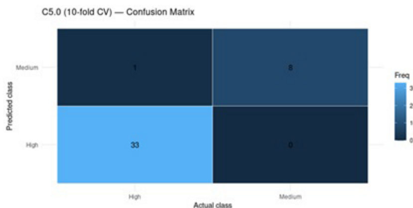
Зураг 1. Алдааны матрицын дүрслэл (Confusion matrix-ийг heatmap).
