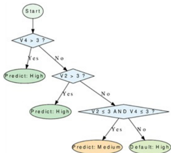
Зураг 3. C5.0 загвараас гарсан сэтгэл ханамжийн ангиллын шийдвэрийн мод.
