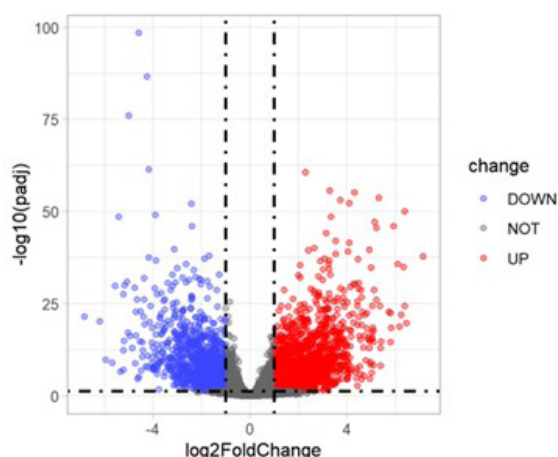
Зураг 1. TCGA өгөгдлийн сан дах ялгаатай экспресслэгдсэн lncRNA шинжилгээ.
