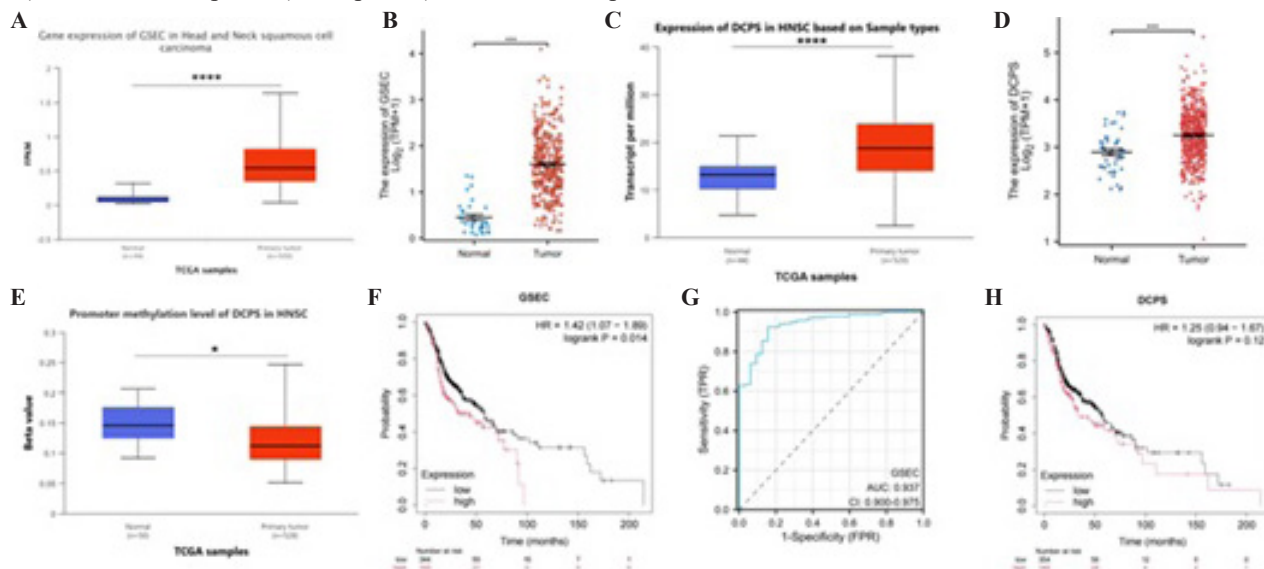
Зураг 3. TXXXЭӨ-гийн эд дэх GSEC ба DCPS -ийн экспресс.
