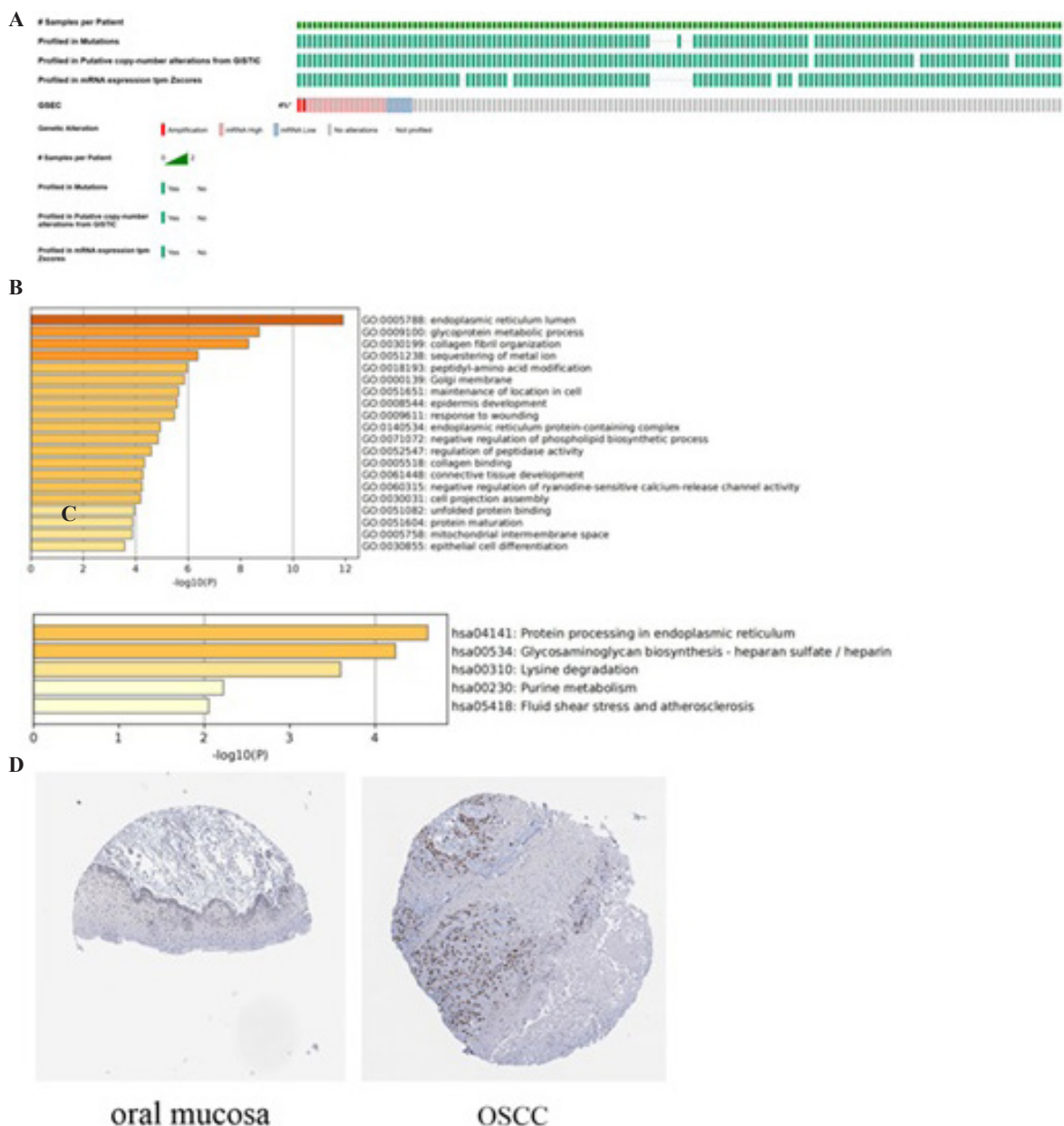
Зураг 4. ТХХХЭӨ дэх GSEC генийн мутаци ба үйл ажиллагааны шинжилгээ.
