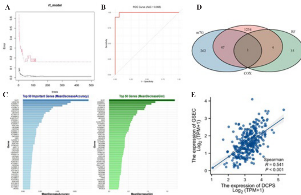
Зураг 2. m7G-тэй холбоотой lncRNA GSEC-ийг тодорхойлсон аргууд.
