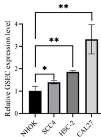
Зураг 5. NHOK ба АХХХЭӨ-гийн шугаман эсүүд дэх GSEC-ийн экспресс
